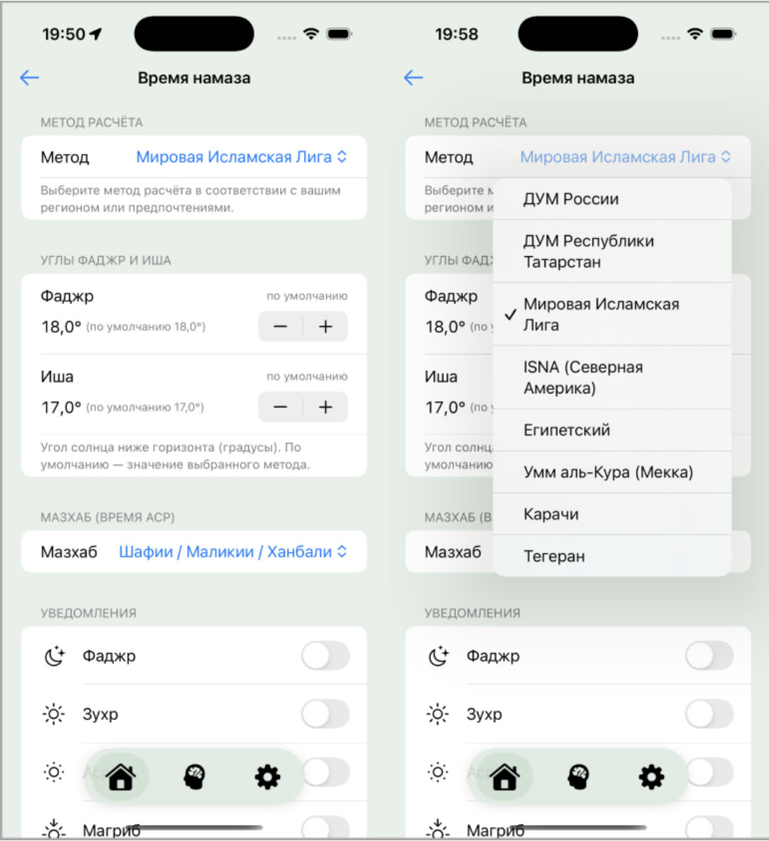
Рис.1.19. Макет экрана настроек времени намаза
