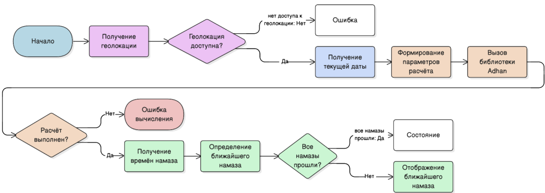
Рис.1.14. Блок-схема алгоритма расчета времени намаза
