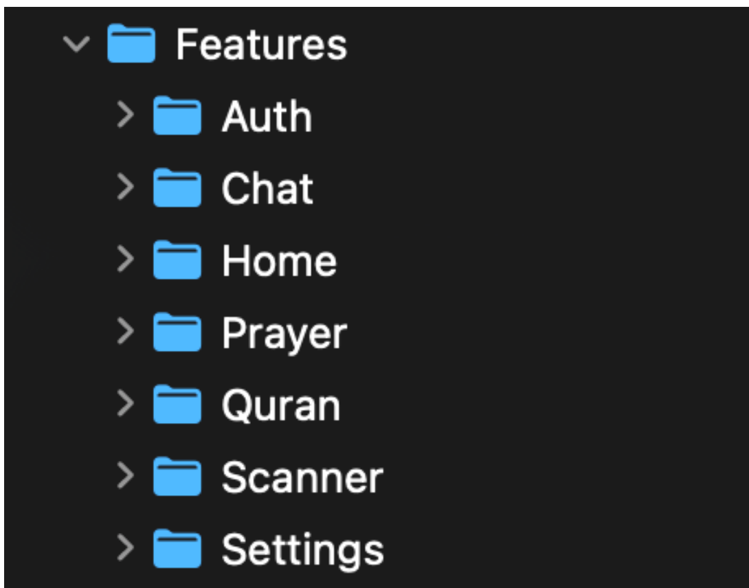
Рис.2.5. Модуль Features
