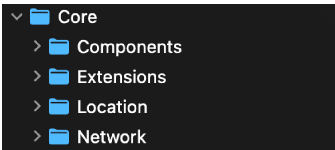
Рис.2.6. Модуль Core
