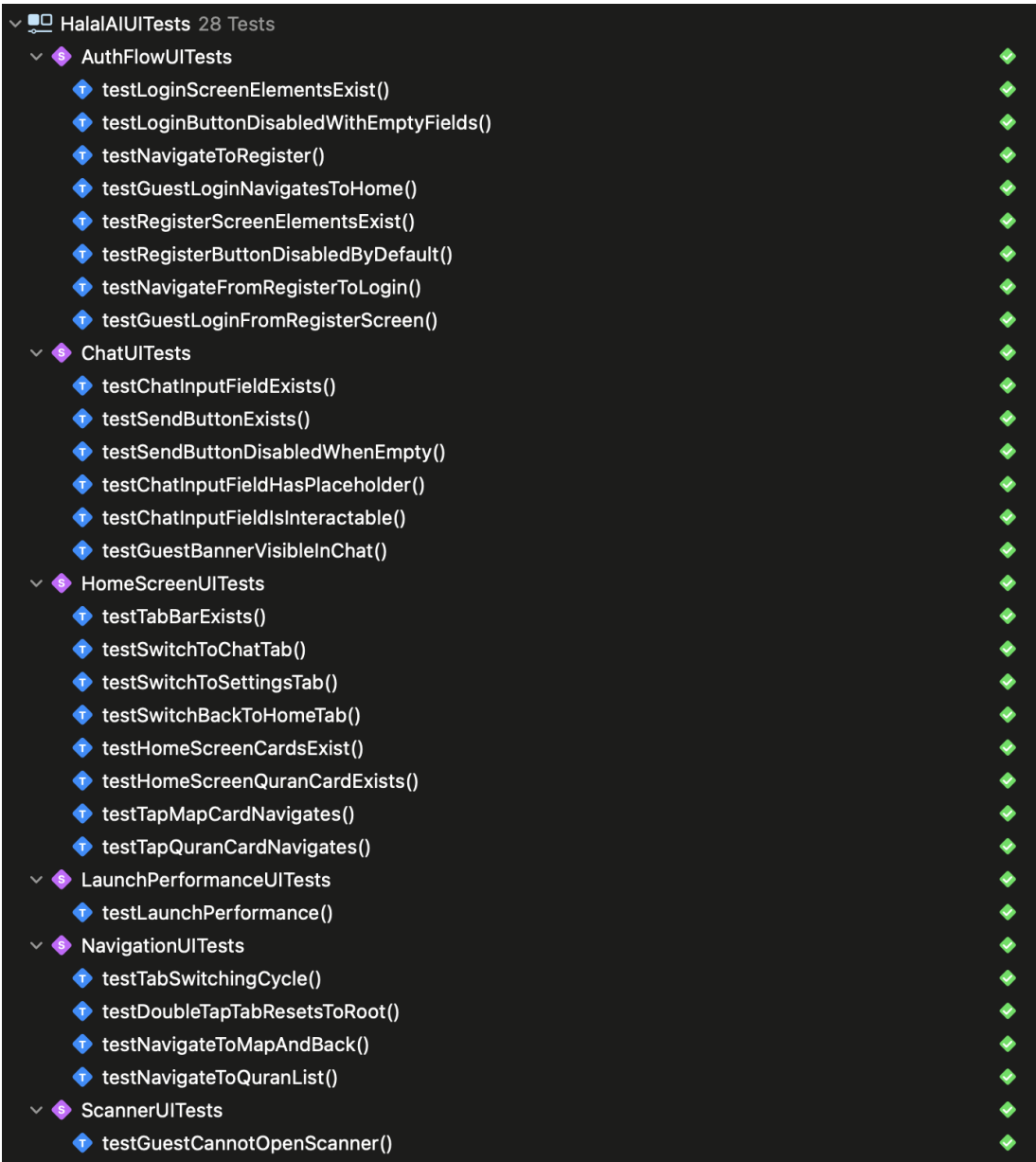
Рис.3.6. iOS UI-тесты
