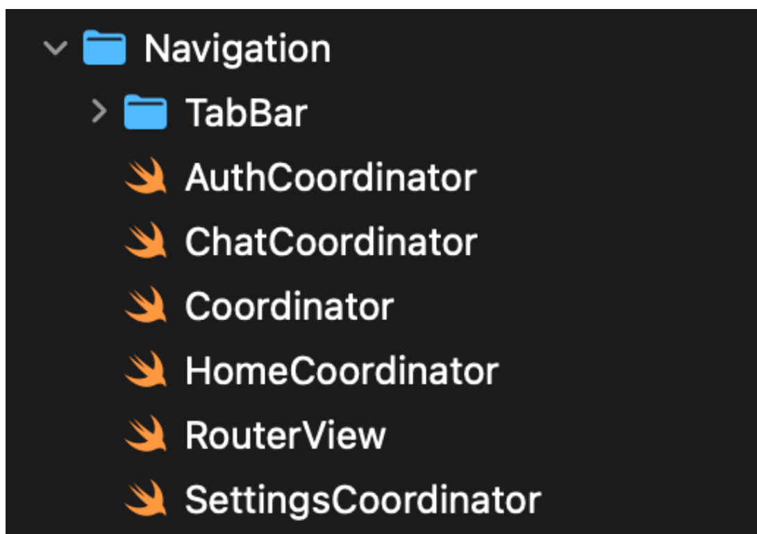
Рис.2.7. Модуль Navigation
