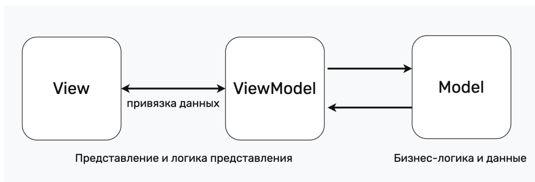
Рис.1.15. MVVM
